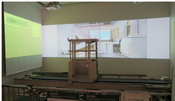
▲振動台BiCURI 地震が起こった時の揺れと建物の中の様子を見ることができます。
